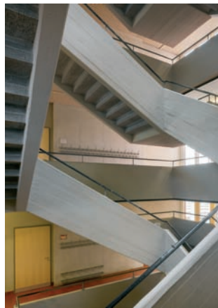
Neue Erdbebenwände in einem ertüchtigten Gebäude wurden architektonisch geschickt integriert (Schulanlage Riedenhalde, Zürich 2007)
